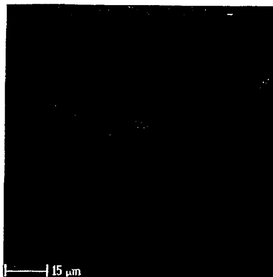
Si-Ka (Spl)
