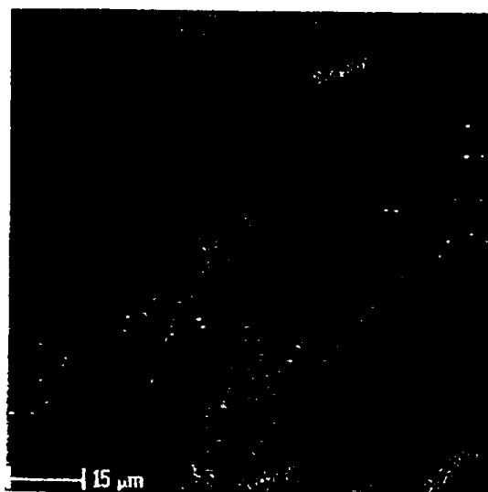
Si-Ka (Spl)
