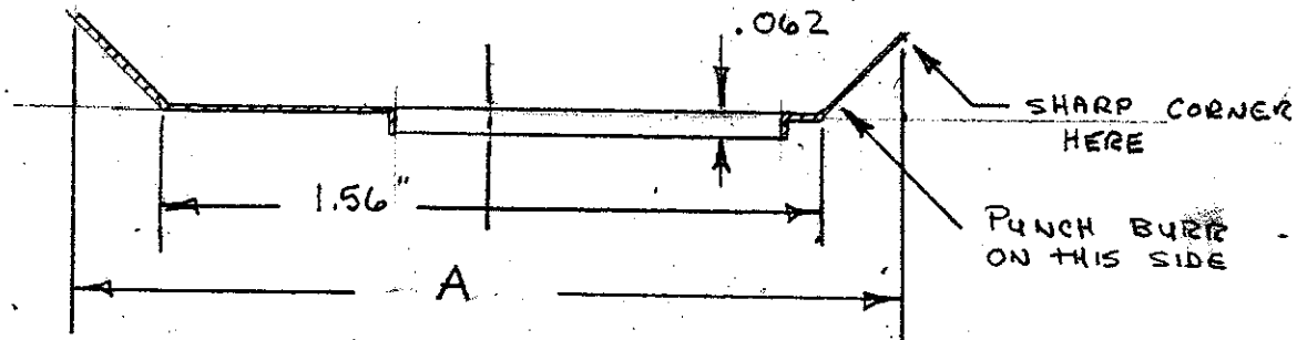
SECT A-A
