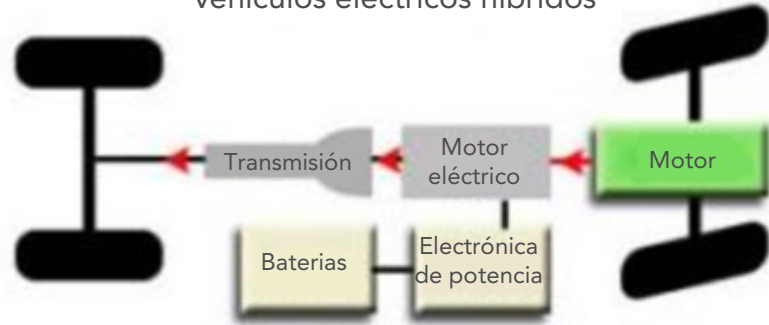
Transmisión paralela de vehículos eléctricos híbridos
