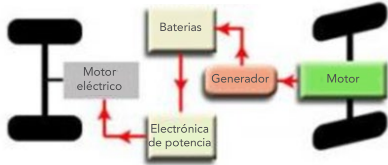
Transmisión de vehículos eléctricos híbridos en serie
